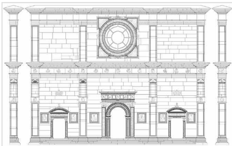
Rilievo della Cattedrale di San Lorenzo, Lugano
